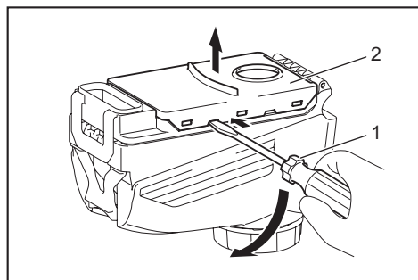
► 1. Destornillador de punta plana 2. Cubierta del filtro
